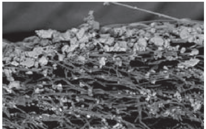
REM Aufnahme eines bestaubten synthetischen Kraftstoff-Filterers
